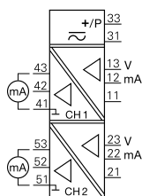
隔离驱动器
